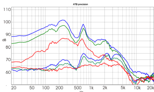
Bild 3.15 Doppelbass V-Anordnung
