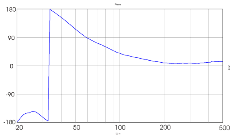
Bild 6.4 Bassreflex
