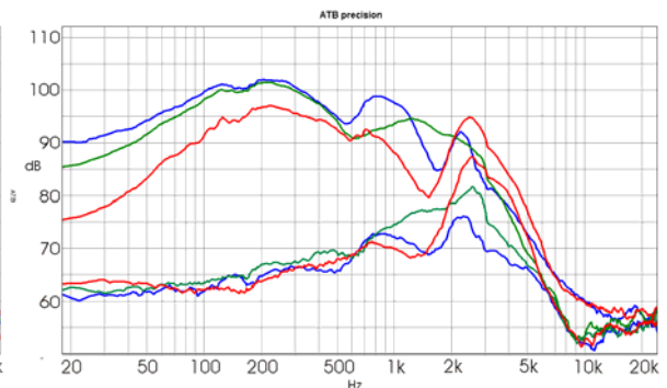
Bild 3.14 Doppelbass nebeneinander
