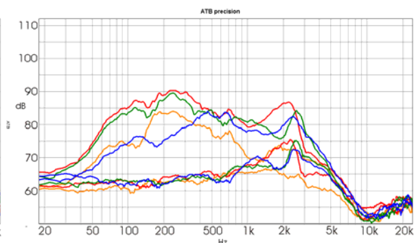
Bild 3.16 Räummessung, Sitzposition
