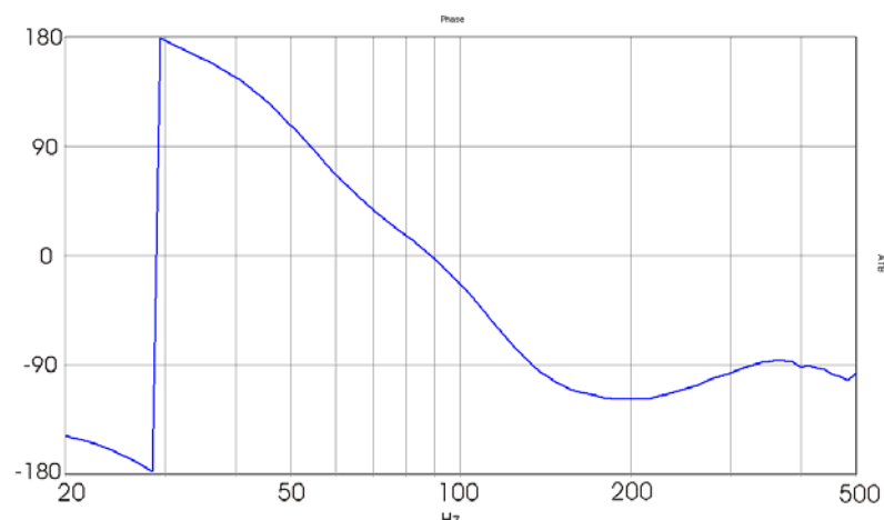
Bild 6.6 Bandpass
