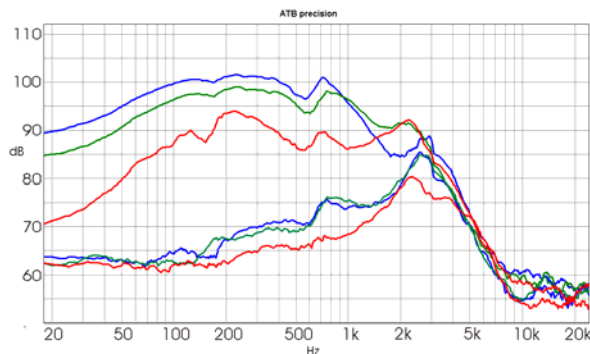
Bild 3.13 Doppelbass übereinander
